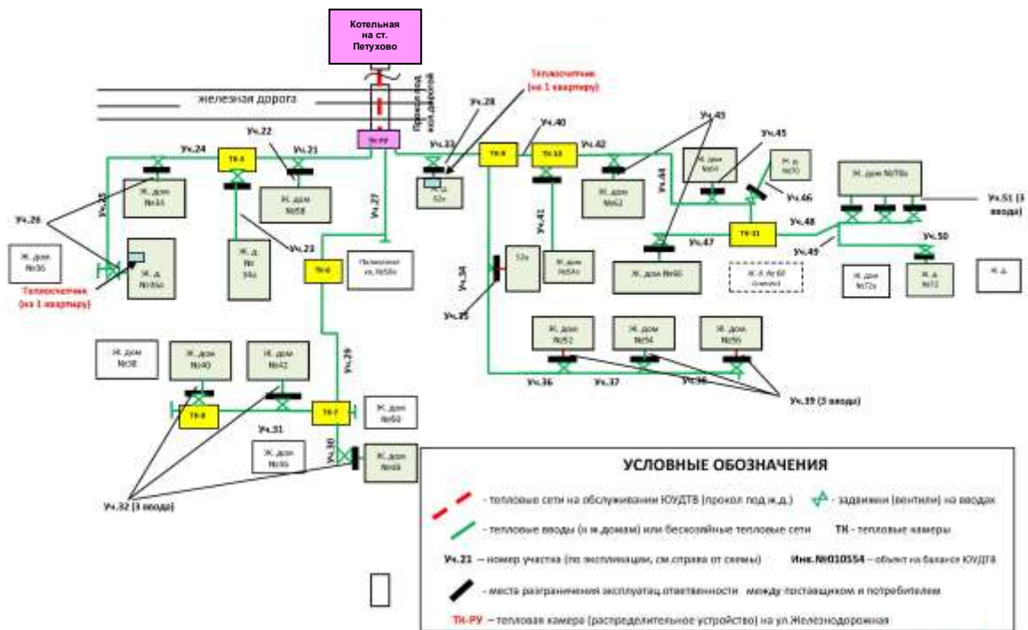
Рисунок 2.15 – Схемы тепловых сетей от котельной ст. Петухово На перспективу изменение зон действия теплоисточников не планируется.
